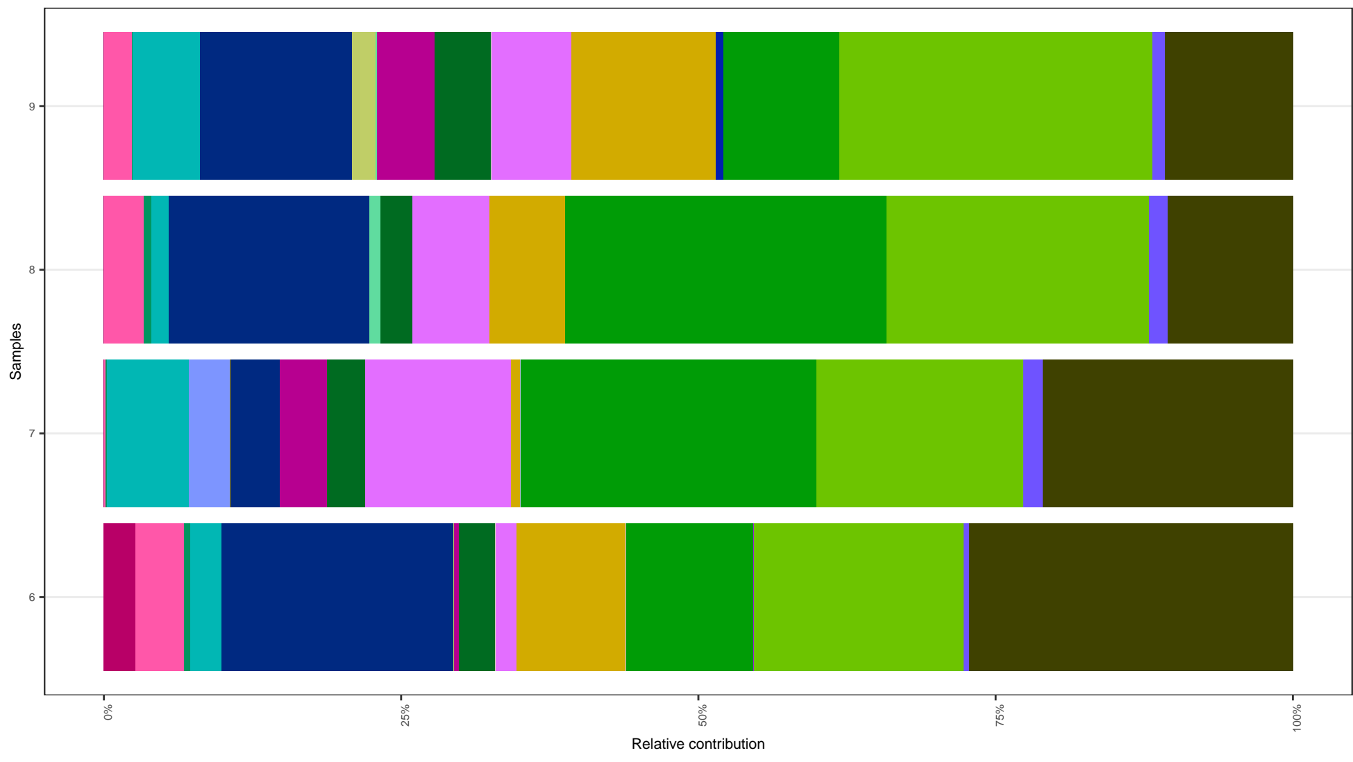
hg38 COSMIC v2
