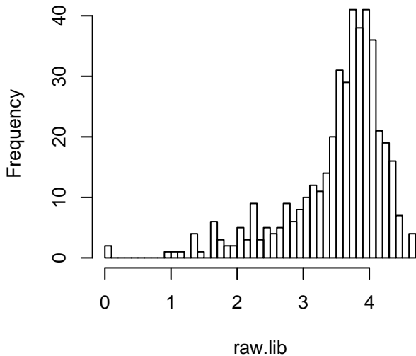
RawData Log10(LibSize)
