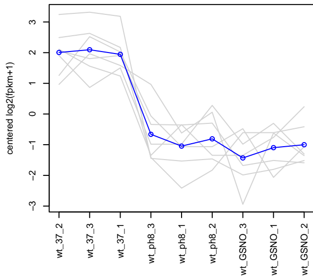
subcluster_2_log2_medianCentered_fpkm.matrix, 7 tran
